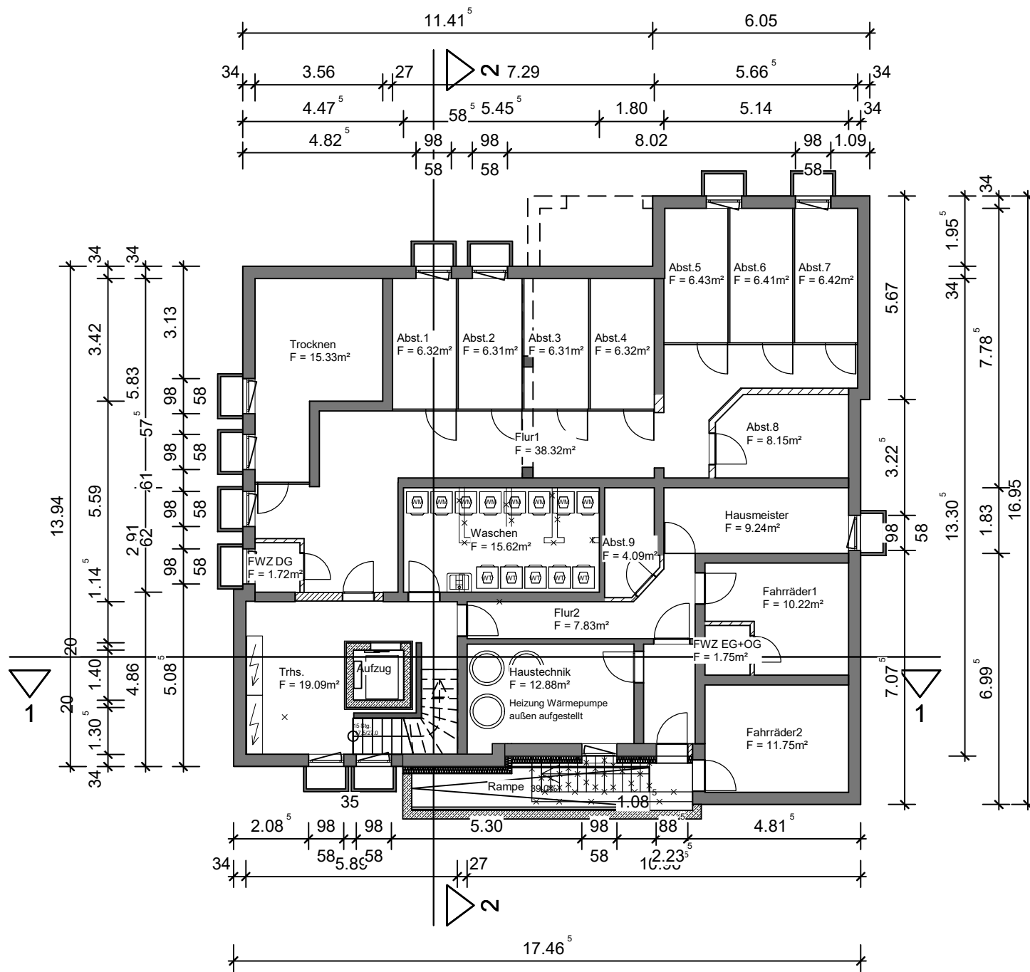
Kellergeschoss unmassstäblich
